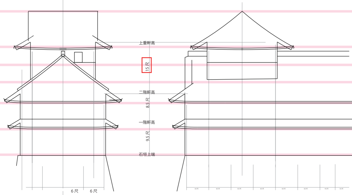
柱間 6 尺
