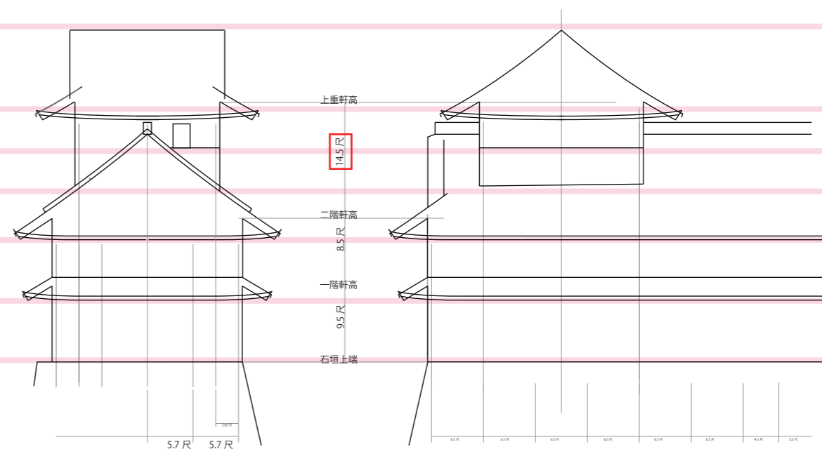
柱間 5.7 尺
